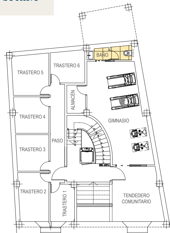
PLANTA SÓTANO
